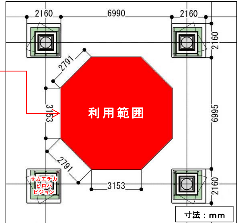
中央スペース 拡大図
