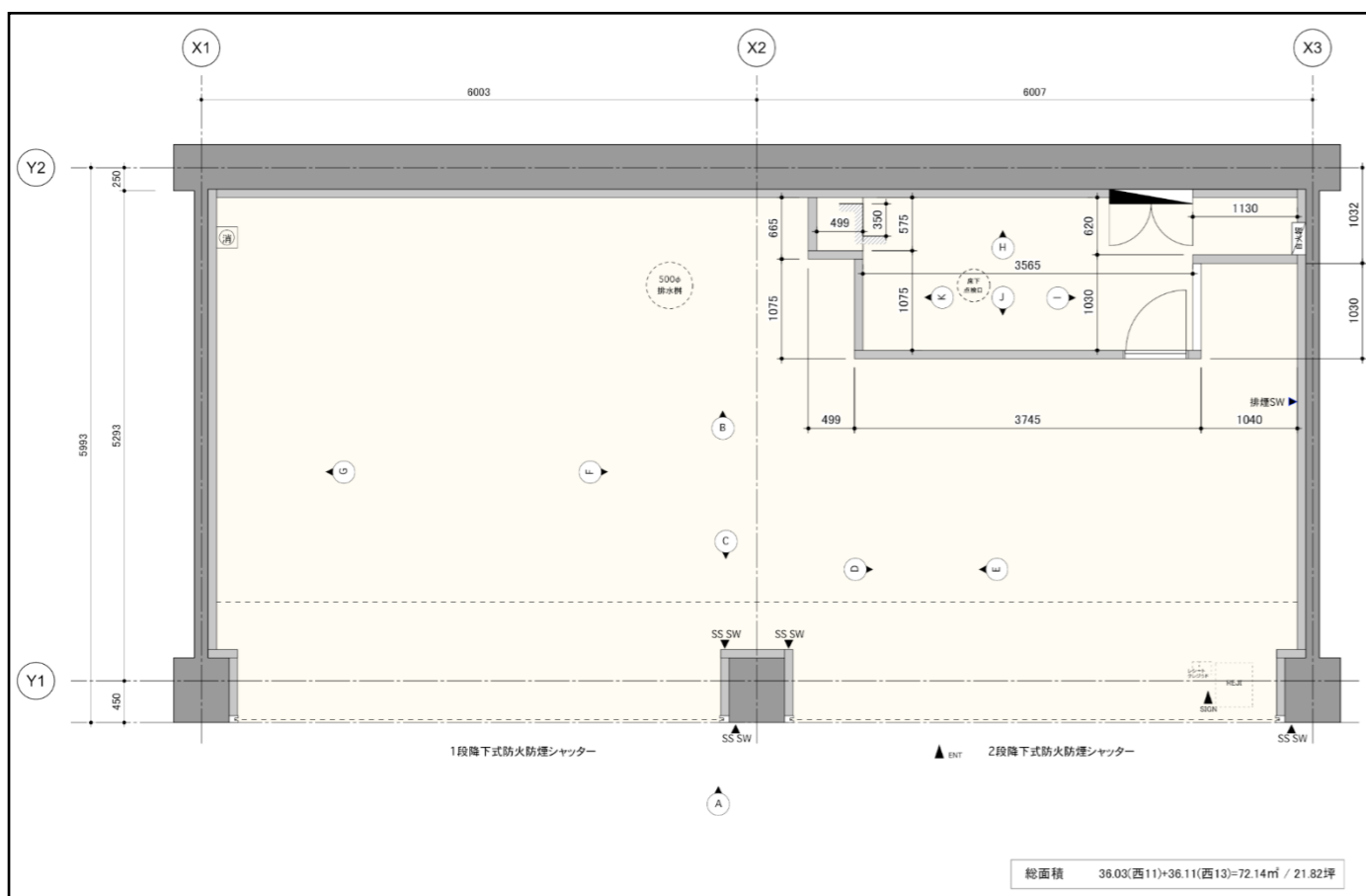
区画図面
